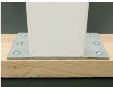
Montageschuh sichtbar verschraubt
