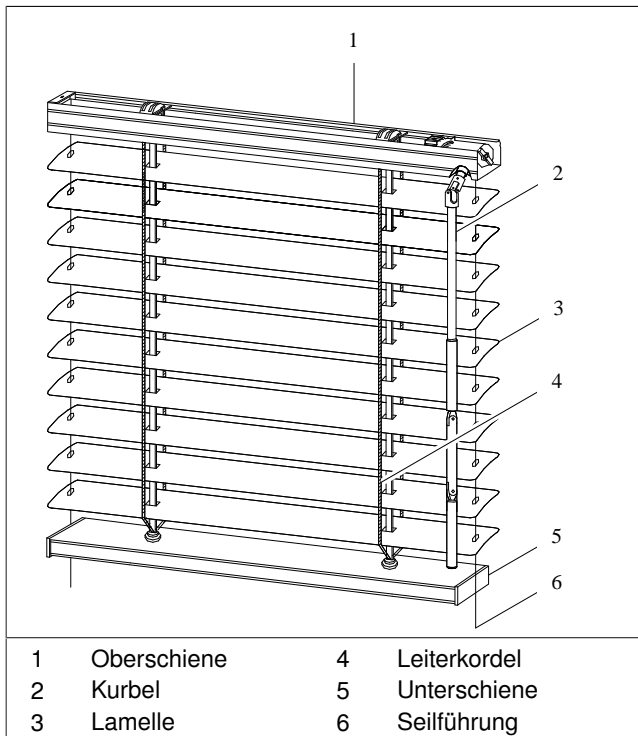
Abb. 1: Teileübersicht Jalousie K50
